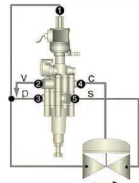
Reductor de presión con solenoide
