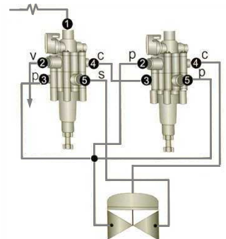
Sostenedor y reductor de presión
