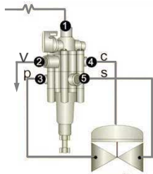
Reductor de presión
